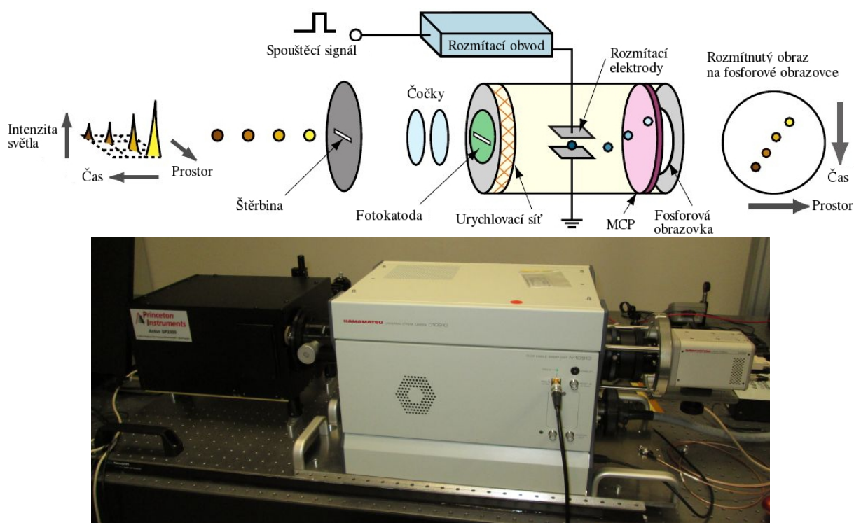
Obrázek 8.8: Nahoře funkční schéma streak kamery (převzato z webu firmy Hamamatsu). Dole fotografie experimentální sestavy, zleva doprava: rozmítací spektrometr, časovací elektronika, iCCD kamera.
