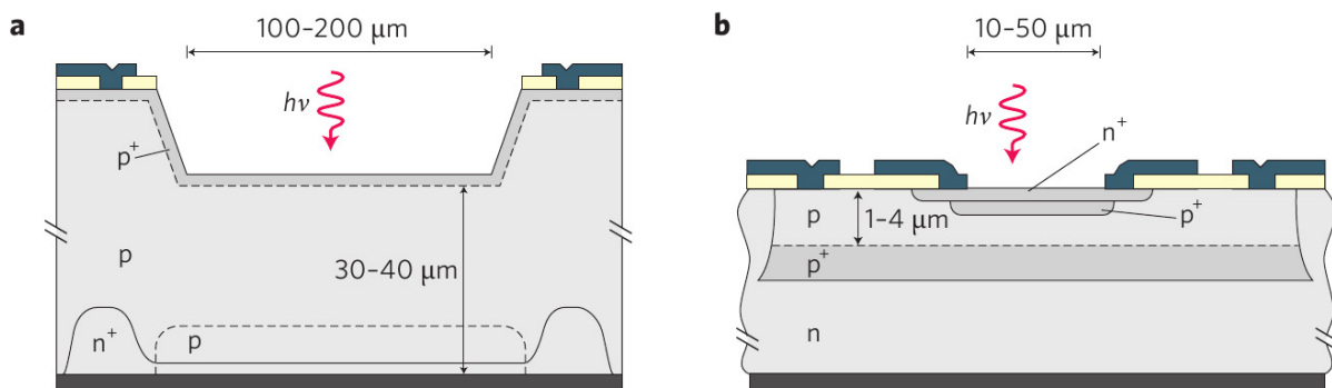
Obrázek 9.4: Průřez čipy jednofotonových lavinových fotodetektorů optimalizovaných a) na kvantovou účinnost, b) na rychlost. Převzato z ref. [26].
