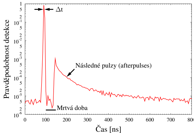
Obrázek 9.1: Histogram normované pravděpodobnosti detekce jednofotonové lavinové diody SPCM-AQ od EG&G Canada.
