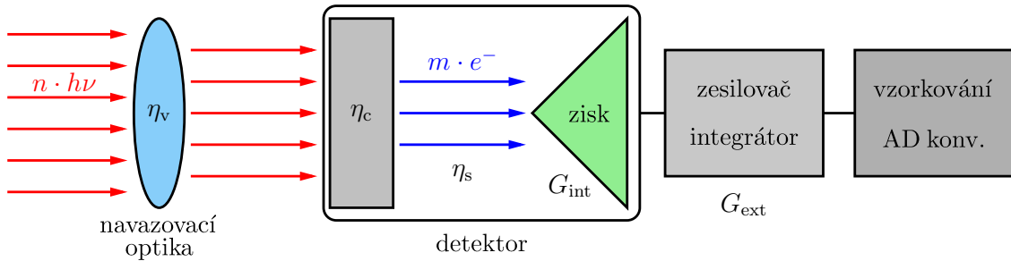
Obrázek 9.2: Funkční schéma detektoru: Počet vstupních fotonů n je redukován účinnostmi navázání \eta_v , konverze \eta_c a sběru primárního náboje \eta_s , počet m fotoelektronů (popř. elektron-děrových párů) je znásoben v procesech vnitřního a vnějšího zesílení faktorem G_{\text{int}} resp. G_{\text{ext}} , vzorkován a digitalizován.
