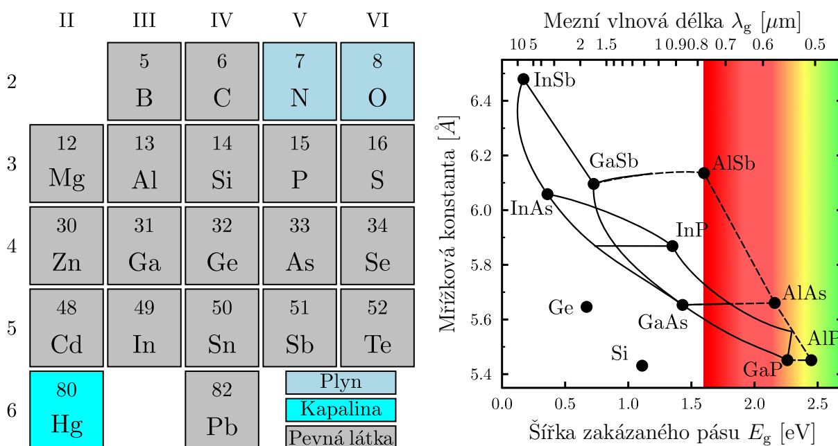
Obrázek 1.7: a) Výsek periodické tabulky prvků. b) Vlastnosti polovodičových materiálů a slitin (převzato a upraveno z [1]).
