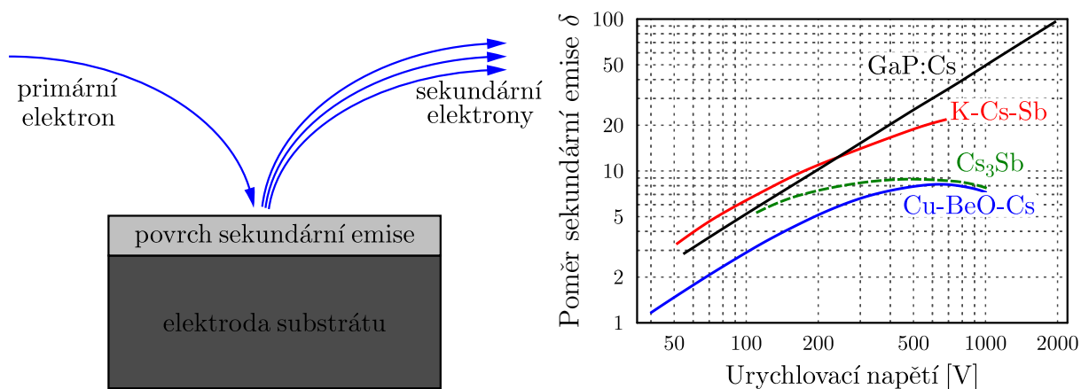
Obrázek 6.5: Vlevo schéma sekundární emise, vpravo závislost poměru sekundární emise \delta na urychlovacím napětí na první dynodu pro různé materiály první dynody (převzato a upraveno z [3]).
