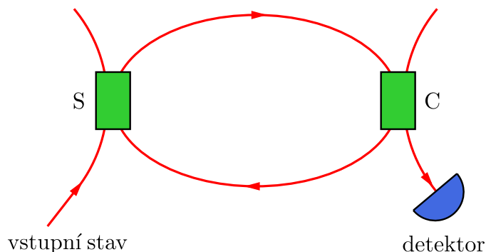
Obrázek 9.12: Schéma smyčkového detektoru, červenou čarou jsou zakreslena optická vlákna, S – optický prepínač, C – dělič optického svazku.
