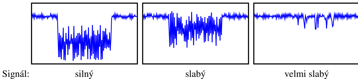
Obrázek 6.7: Výstup fotonásobiče pro různě silné signály.
