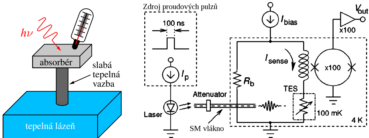
Obrázek 9.9: Mikrokalorimetr na hraně supravodivosti, vlevo – funkční schéma, vpravo – elektrické zapojení (převzato a upraveno z [31]).
