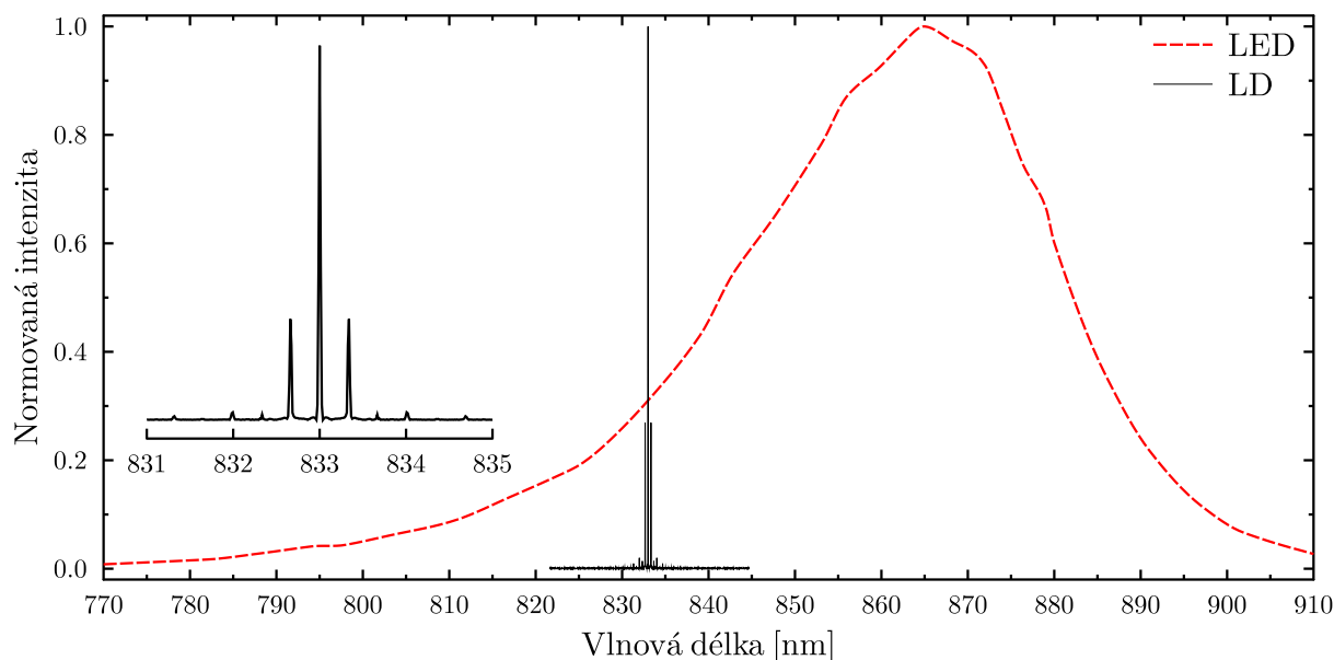
Obrázek 2.7: Spektrum laserové diody OZ Optics (LD) s centrální vlnovou délkou 816 nm (spektrum spočteno jako FFT autokorelační funkce) v porovnání s LED. Spektrum plynového laseru by bylo při tomto rozlišení \delta -funkcí.
