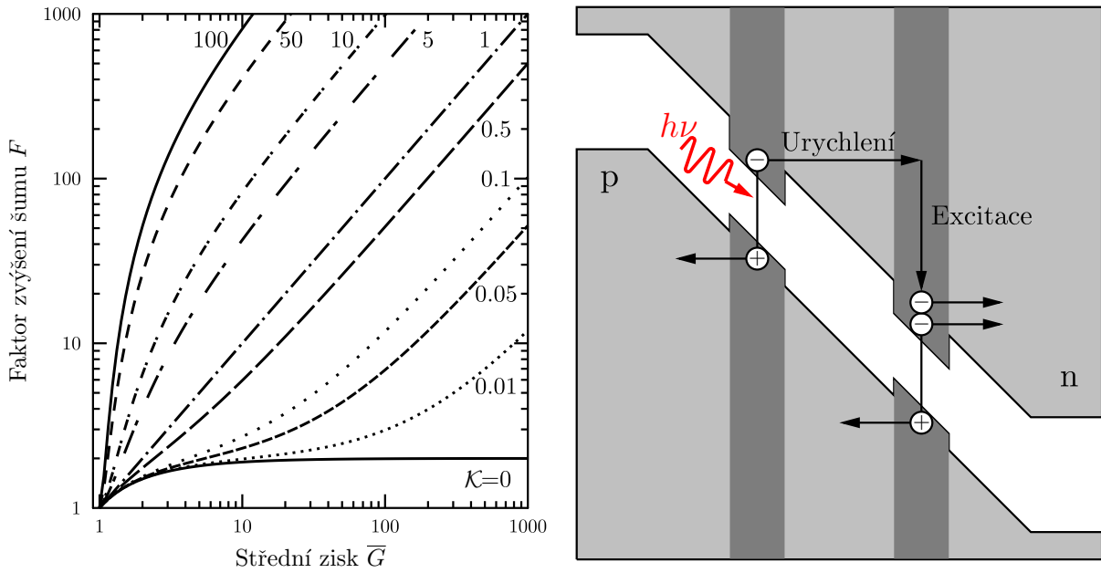
Obrázek 5.4: Vlevo závislost faktoru zvýšení šumu F na středním zisku pro různé ionizační poměry v detektoru s elektronovou multiplikací, vpravo schéma APD s heterostrukturou.
