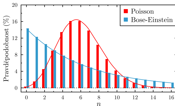
Obrázek 2.1: Pravděpodobnosti počtu n fotonů v pulzu u Boseova-Einsteinova a Poissonova rozdělení.
