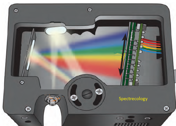
Obrázek 7.25: Schéma spektrometru Flame od firmy Ocean Optics. Difrakční mřížka je umístěna v otočné montáži. Po zafixování rotace dvěma šroubky je třeba spektrometr nakalibrovat. Převzato z webu Ocean Optics [19].
