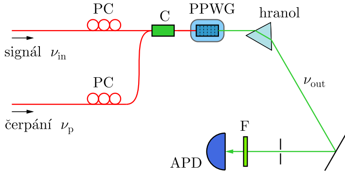
Obrázek 9.5: Schéma detektoru APD s upkonverzí, červenou čarou jsou zakreslena optická vlákna, PC – polarizační kontrolér, C – vláknový slučovač, PPWG – periodicky pólovaný vlnovod, F – spektrální filtr.
