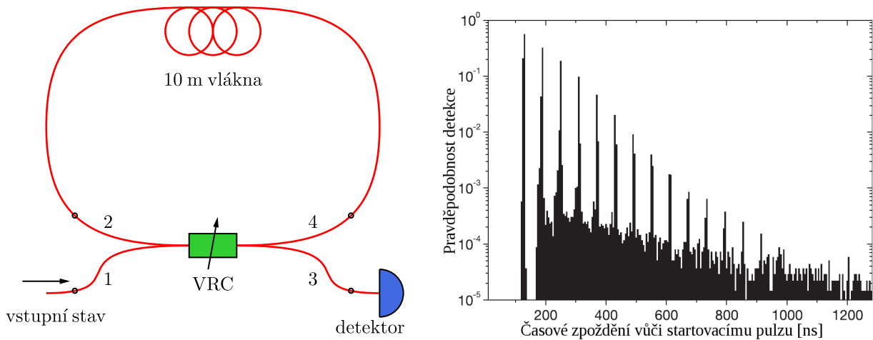
Obrázek 9.13: Vlevo schéma smyčkového detektoru s nevyváženým děličem SVR, vpravo histogram detekčních událostí z tohoto detektoru (převzato a upraveno z [37]).
