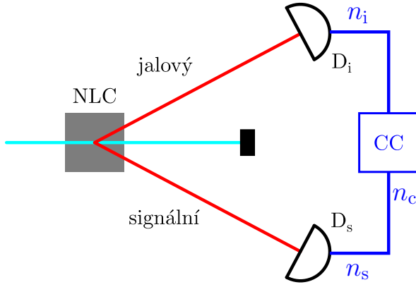
Obrázek 9.3: Určení kvantové účinnosti detektoru pomocí spontánní parametrické sestupné konverze v nelineárním krystalu.
