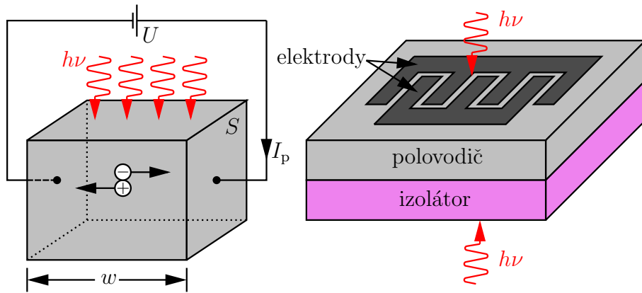
Obrázek 4.1: Schéma elektrického obvodu polovodičového detektoru.
