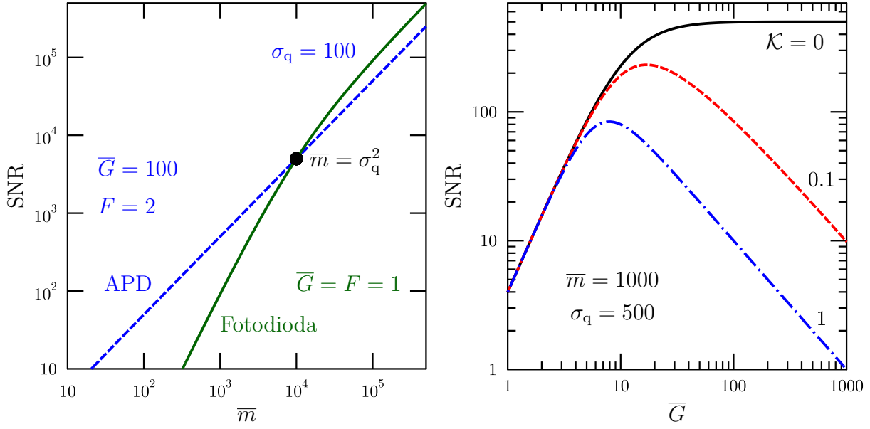
Obrázek 5.5: Závislost SNR na středním počtu fotoelektronů \bar{m} (vlevo) a na středním zisku \bar{G} (vpravo).
