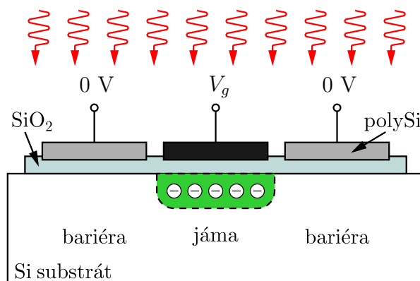
Obrázek 7.3: Schéma jednoho pixelu CCD se třemi kontakty, které upravují potenciál potřebný pro vytvoření potenciálové jámy (zelená oblast) pro udržení a následný posun generovaných fotoelektronů.
