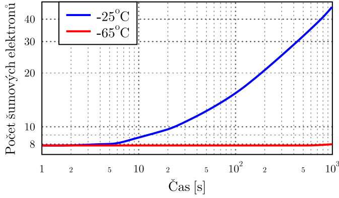
Obrázek 7.7: Závislost šumu v podobě termálně excitovaných elektronů na čase a teplotě (převzato a upraveno z [?]).
