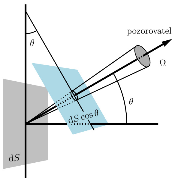
Obrázek 1.3: Geometrické aspekty výpočtu záře tělesa.
