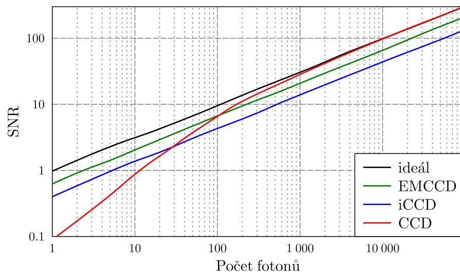
Obrázek 8.10: Srovnání kamer podle poměru signálu k šumu (podle Andor).
