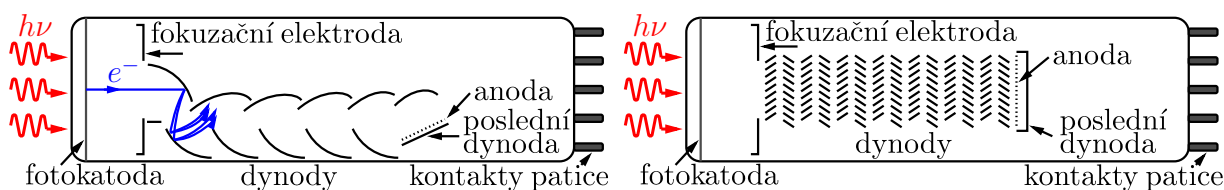
Obrázek 6.15: Lineárně fokusovaný (vlevo) a žaluziový (vpravo) typ fotonásobiče.
