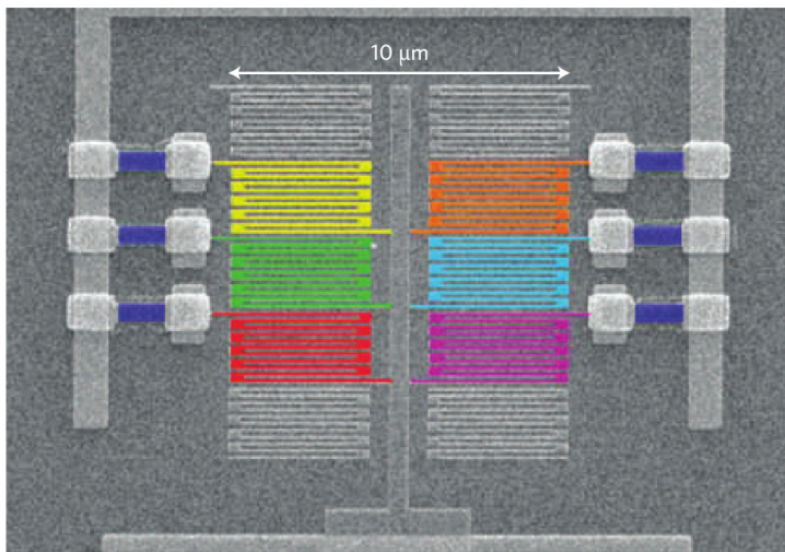
Obrázek 9.10: Multiplex šesti supravodivých nanovláken. Pro názornost byl obrázek barevně upraven (převzato z [32]).
