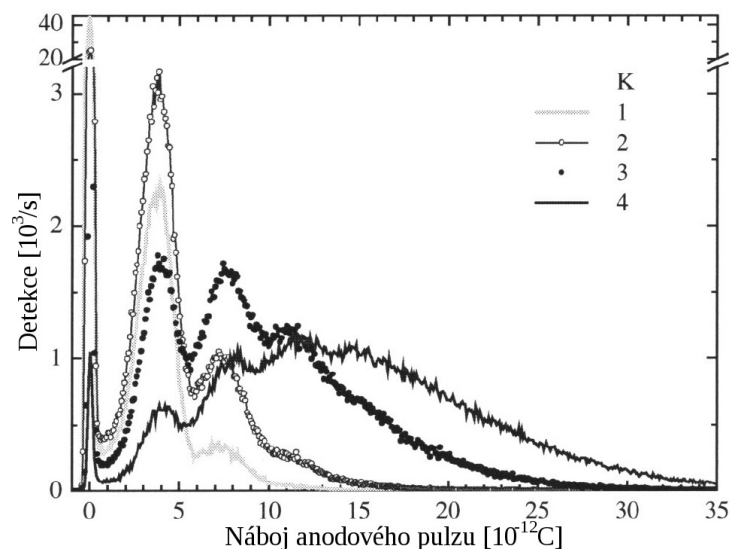
Obrázek 9.6: Rozložení velikosti pulzů ze speciálního fotonásobiče popsaného v textu odpovídající různým počtům fotonů (převzato z [29]).
