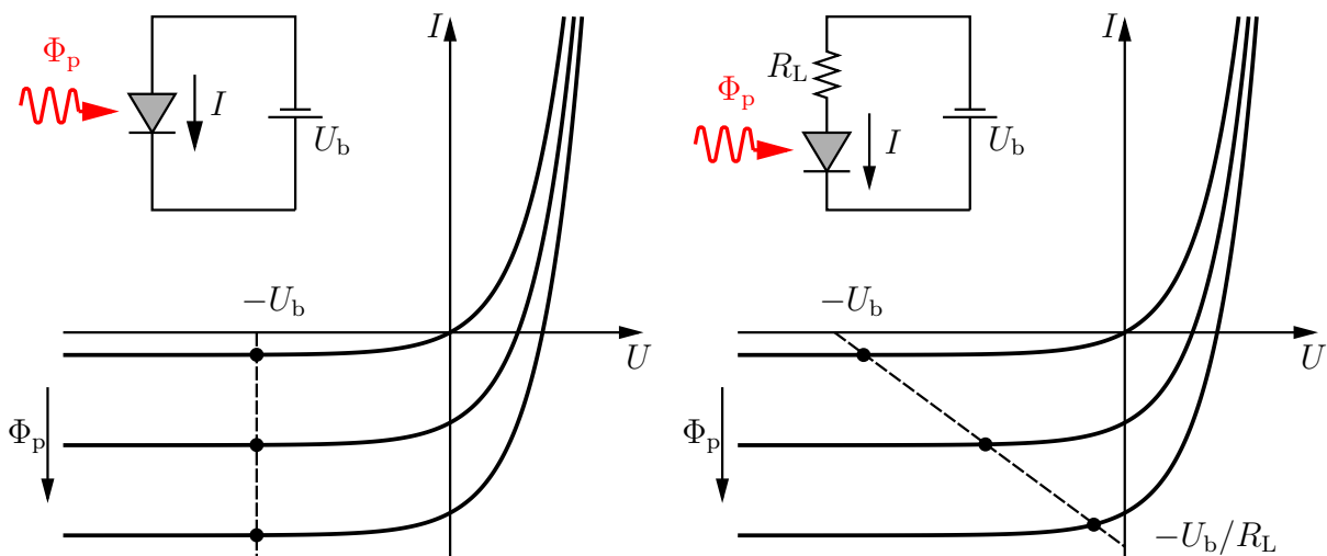
Obrázek 4.6: Průběh voltampérové závislosti pro elektrické zapojení se závěrným napětím a) bez a b) s odporem v sérii.
