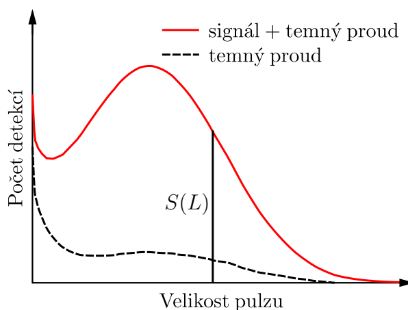
Obrázek 6.8: Histogram velikosti proudových pulzů na výstupu fotonásobiče (převzato a upraveno z [3]).
