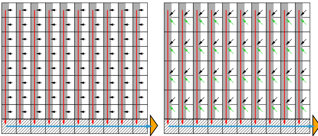
Obrázek 7.13: Vyčítání CCD s Interline transfer архитектурou, vlevo progresivní a vpravo prokládaný způsob.
