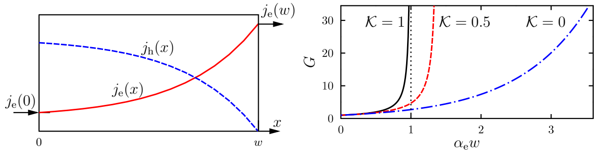
Obrázek 4.12: Závislost a) proudové hustoty elektronů ( j_e ) a děr ( j_h ) na poloze v multiplikační oblasti, b) závislost zisku pro hodnoty \mathcal{K} = 1, 0.5 a 0 .
