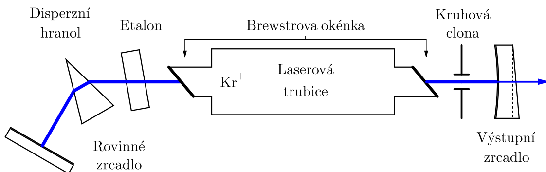
Obrázek 2.3: Schéma plynového laseru, aktivní prostředí tvoří kryptonový plyn čerpaný elektrickým polem. Kruhová clona vymezuje prostorové módy, které mohou vzniknout v rezonátoru délky d tvořeného zrcadly. Náklon disperzního hranolu určuje vlnovou délku laserového záření, etalonu tloušťky d_1 navíc vymezuje pouze jeden frekvenční mód.
