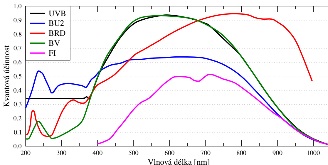
Obrázek 7.24: Kvantová účinnost různých senzorů kamery iKon (podle specifikace Andor [20]).
