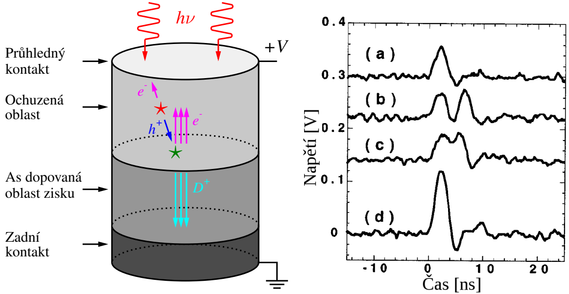
Obrázek 9.8: Vlevo – schéma VLPC, vpravo – časové překrytí dvou jednofotonových událostí (převzato a upraveno z [30]).
