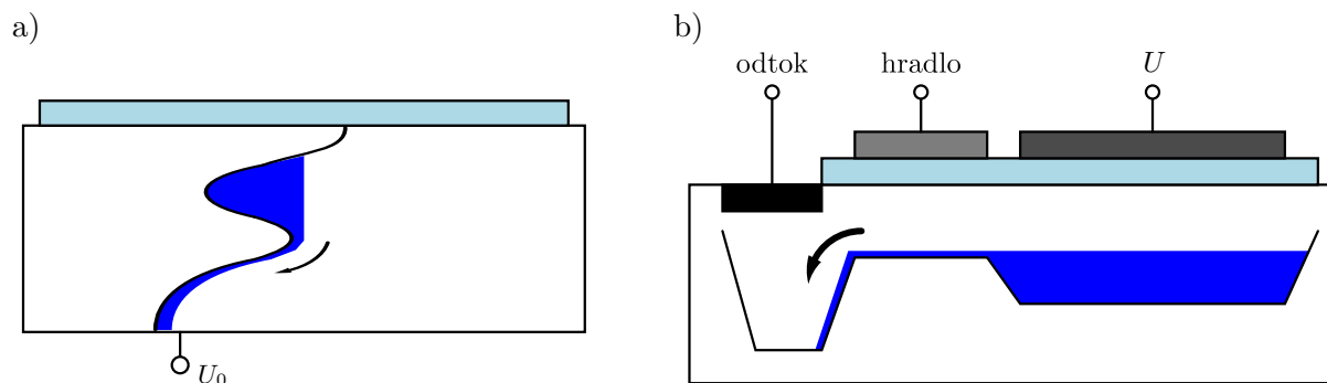
Obrázek 7.19: Schémata obvodu přetečení (odtokového kanálku): a) vertikální (VOD), b) laterální (LOD).
