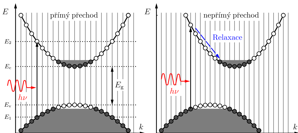
Obrázek 1.6: Tvar energetických pásů v závislosti na velikosti vlnového vektoru v případě přímého přechodu (vlevo) a nepřímého přechodu (vpravo).
