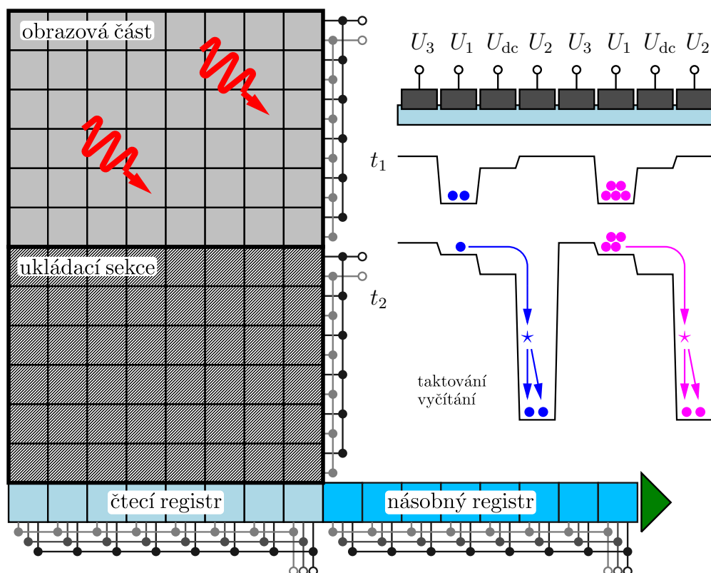
Obrázek 8.1: Schéma elektronové multiplikace EM-CCD. Vpravo nahoře je schéma kontaktů a profil napětí na kontaktech během multiplikačního přesunu do násobného registru.
