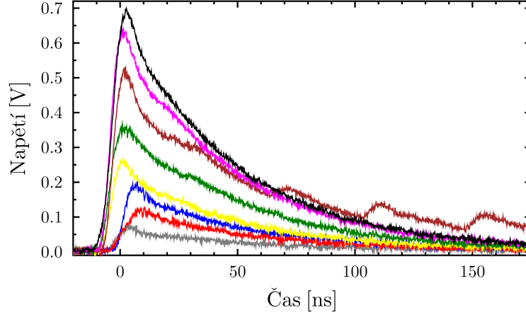
Obrázek 9.16: Velikost výstupního napětí z MPPC (Hamamatsu C11208) v závislost na počtu zaregistrovaných fotonů.
