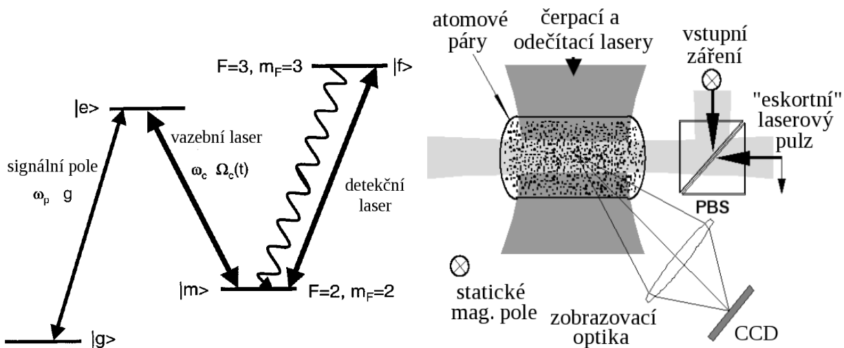
Obrázek 9.11: Vlevo – energetické hladiny atomu Cs, vpravo – schéma detektorů založeného na excitaci atomů (převzato a upraveno z [33]).
