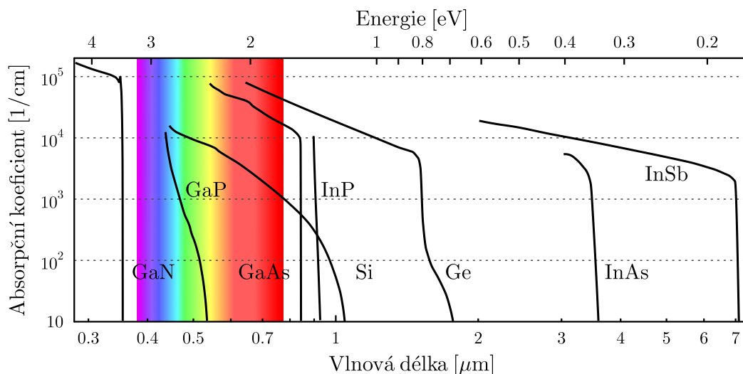
Obrázek 1.10: Absorpční koeficient v závislosti na vlnové délce (energii) fotonu pro různé materiály (převzato a upraveno z [1]).
