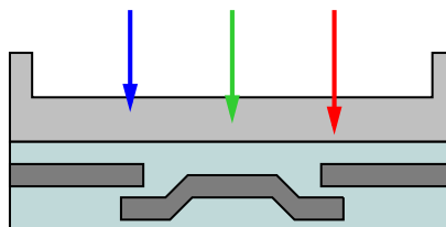
Obrázek 7.5: Schéma jednoho pixelu tenčeného CCD čipu se zadním osvětlením.
