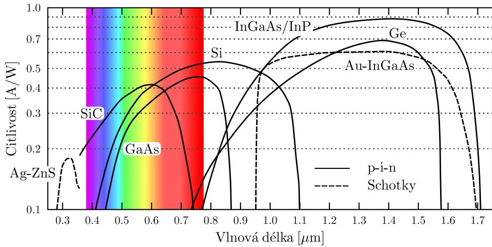
Obrázek 1.11: Citlivost různých materiálů v závislosti na vlnové délce (převzato a upraveno z [1]).
