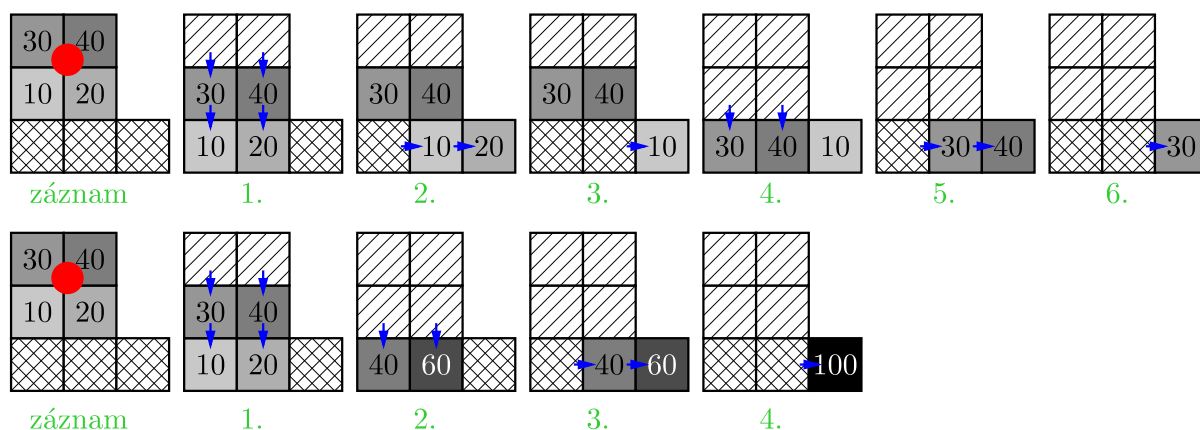
Obrázek 7.10: Porovnání rychlosti vyčítání informace pro nesdružené (horní řada) a 2×2 hardwarově sdružené (spodní řada) pixely.
