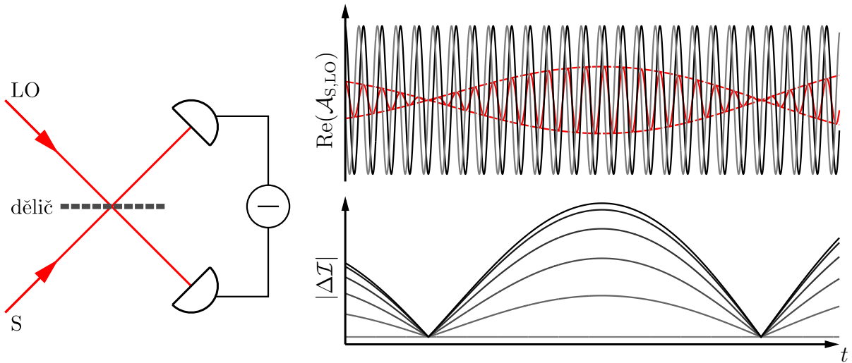
Obrázek 3.12: Vlevo schéma homodynní detekce s měřením rozdílu výstupních fotoproudů. Vpravo nahoře průběh komplexních amplitud signálu (S, červeně) a lokálního oscilátoru (LO, černá a šedá), vpravo dole průběh rozdílu intenzit v závislosti na změně fáze \varphi_{LO} .
