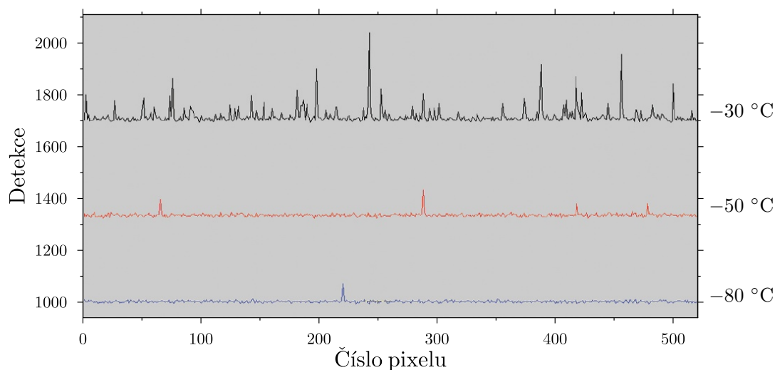
Obrázek 8.4: Šum EM-CCD detektoru v závislosti na teplotě. Jak je zřejmé, pro snížení šumu je nutné chlazení detekčního čipu pomocí více stupňového Peltierova článku na teplotu menší než −80 °C.
