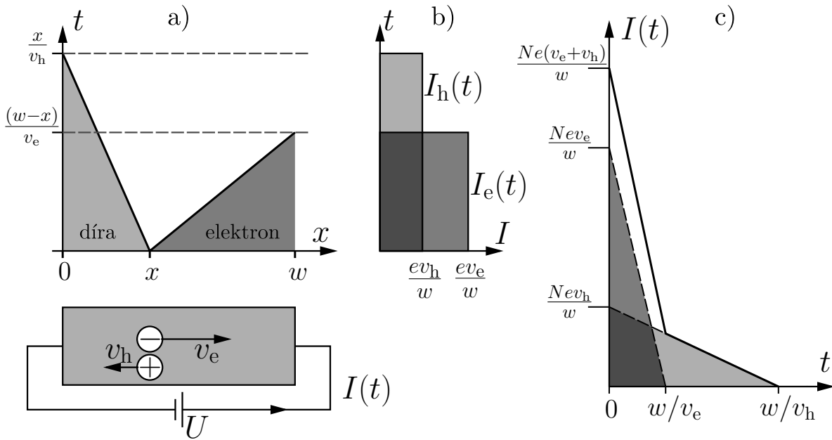
Obrázek 1.12: a) Schéma zobrazující dobu průchodu elektron-děrového páru materiálem fotodetektoru. b) Závislost elektrického proudu na čase způsobeného jedním párem nosičů po absorpci fotonu na pozici x . c) Průběh elektrického proudu v závislosti na čase v případě dopadu fotonu v náhodném místě detektoru.
