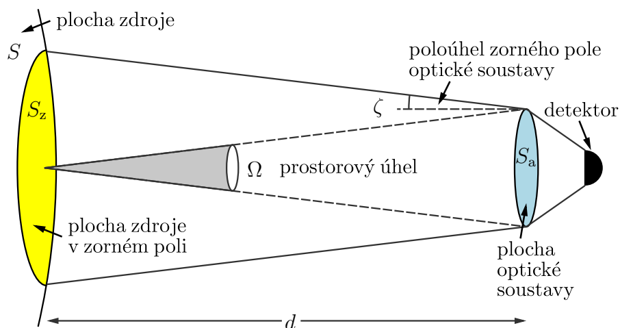
Obrázek 1.5: Geometrické aspekty přenosu optického výkonu.
