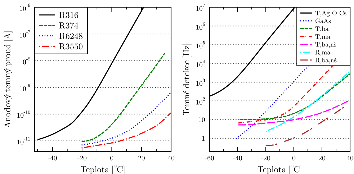
Obrázek 6.12: Vlevo závislost anodového temného proudu, vpravo počet temných detekcí při fotonovém čítání v závislosti na teplotě několika fotonásobičů firmy Hamamatsu [3]. T/R značí transmisní/reflexní fotokatodu, ba, popř. ma bialkalickou a multialkalickou slitinu fotokatody, nš značí nízkošumovou úpravu.
