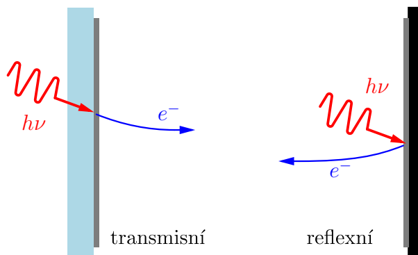
Obrázek 6.3: Funkční schéma průběhu fotoefektu v případě transmisní a reflexní fotokatody.
