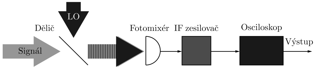
Obrázek 3.10: Schéma heterodynního detektoru, LO značí lokální oscilátor.
