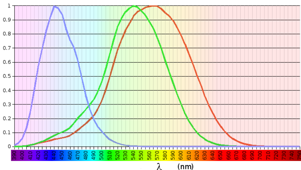
Obrázek 3.3: Relativní spektrální citlivost B, G a R čípků (převzato z [8]).
