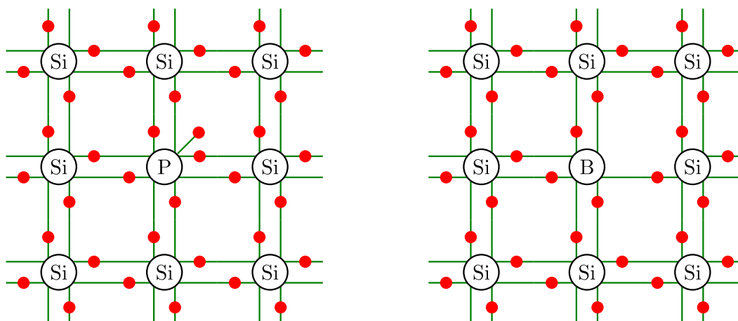
Obrázek 1.8: Znázornění vazeb atomů v mřížce dopovaného polovodiče, vlevo n-typ s přebývajícím elektronem, vpravo p-typ s chybějícím elektronem.
