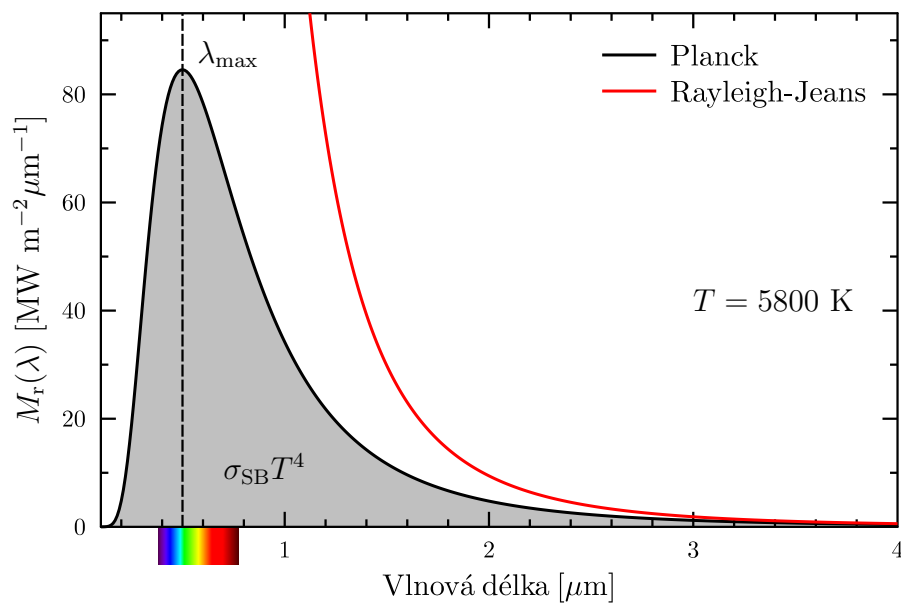
Obrázek 1.4: Vyzařovací charakteristika Slunce podle Rayleighova-Jeansova a Planckova zákona.
