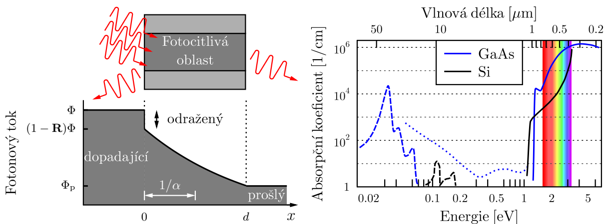
Obrázek 1.9: a) Změna velikosti fotonového toku při průchodu materiálem. b) Závislost absorpčního koeficientu na energii (vlnové délce) fotonu odpovídající různým procesům (převzato a upraveno z [1]). Plná čára značí mezipásové přechody, přerušovaná čára fononovou absorpci a tečkovaná absorpci na volných nosičích.
