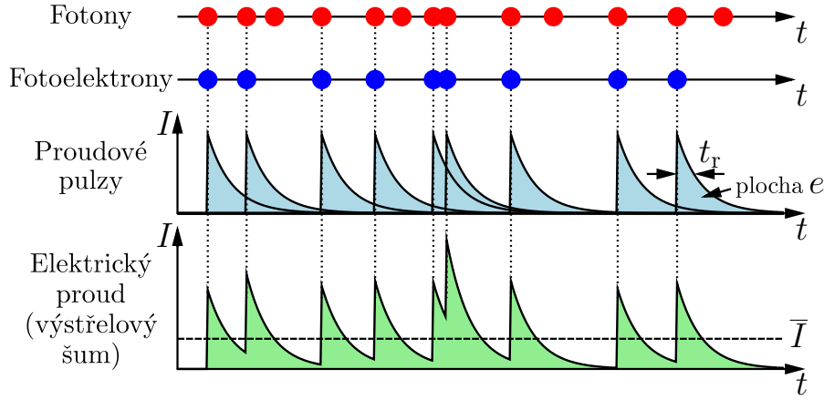
Obrázek 5.3: Průběh elektrického proudu v závislosti na dopadajících fotonech.
