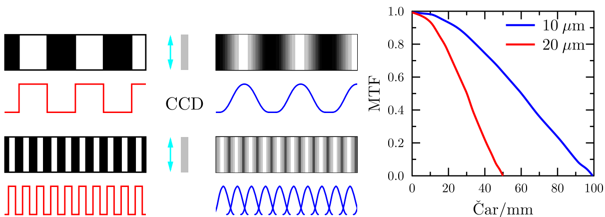
Obrázek 7.8: Vlevo testovací obraz obsahující mřížky o dvou různých prostorových frekvencích. Uprostřed záznam mřížky pomocí kamery, hrany se v důsledku nedokonalého zobrazení a záznamu zahladí, pro větší prostorové frekvence se začínou jednotlivé vrypy překrývat. Vpravo funkce přenosu kontrastu pro senzory s velikostí pixelu 10 a 20 \mu\text{m} (podle Andor).
