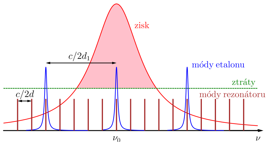
Obrázek 2.4: Faktory ovlivňující emisní spektrum laseru s rezonátorem o délce d , popř. s etalonem tloušťky d_1 .
